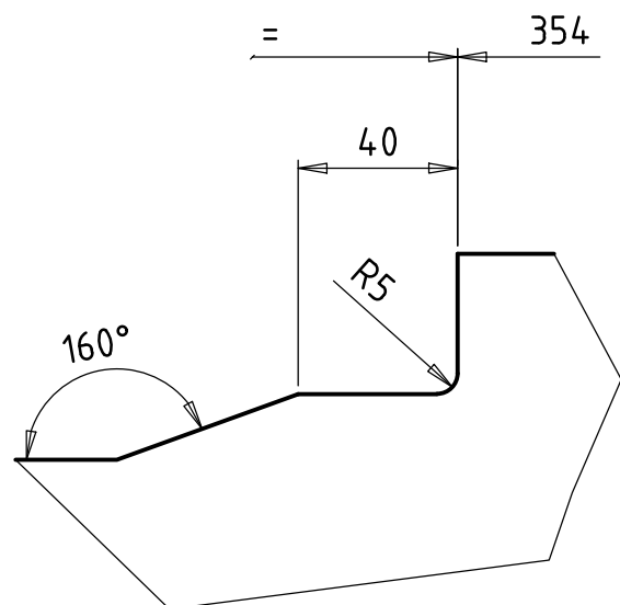
PART. A scala 1:2
